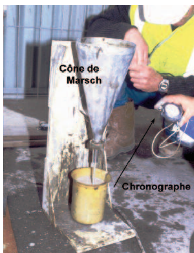
Photo n° 43 : mesure du temps d'écoulement (viscosité) d'un coulis d'injection au cône de March (crédit photo Parexlanko)
