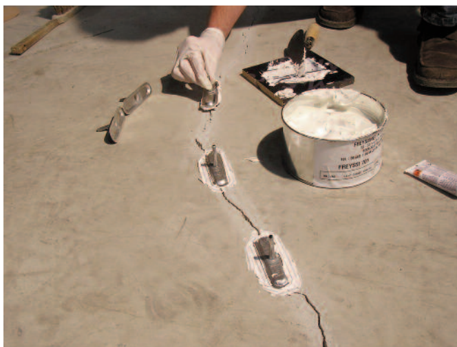
Photo n° 9 : fissure en cours de cachetage (crédit photo Freyssinet)
