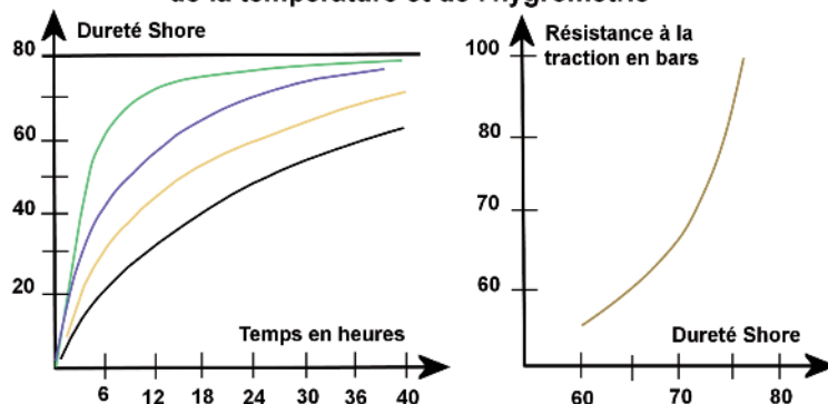
Figure n° 16 : courbes d'évolution de la polymérisation en fonction de la température et de l'hygrométrie de l'air
