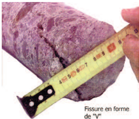
Photo n° 31 : fissure en forme de « V » ouverte mais de faible profondeur (crédit photo Poinéau)
