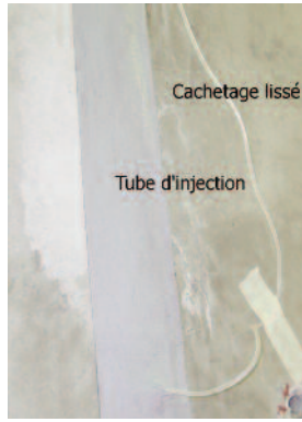
Photo n° 32 : cachetage en bande et lissé (crédit photo Poineau)
