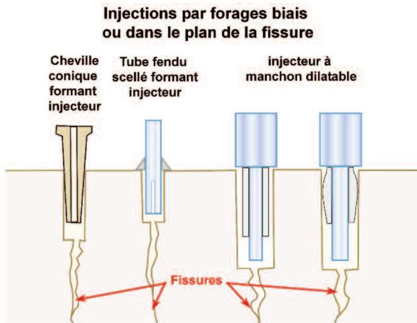
Figure n° 7 : différents modèles d'injecteurs forés
