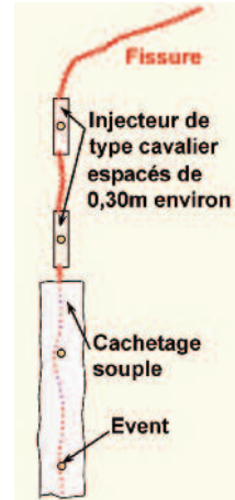
Figure n° 9 : détail de mise en place d'événements collés
