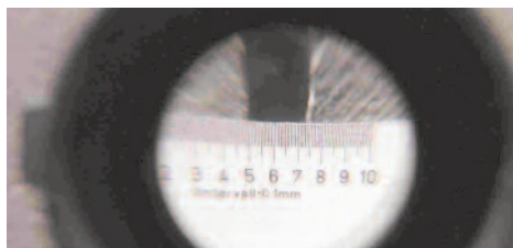
Photo n° 23 : mesure de l'ouverture apparente d'une fissure au moyen d'un compte-fils (crédit photo Freyssinet)
