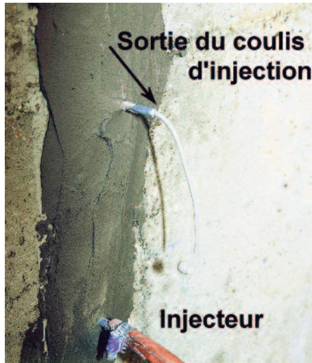
Photo n° 45 : contrôle de la sortie du coulis d'injection aux événements (crédit photo Parexlanko)
