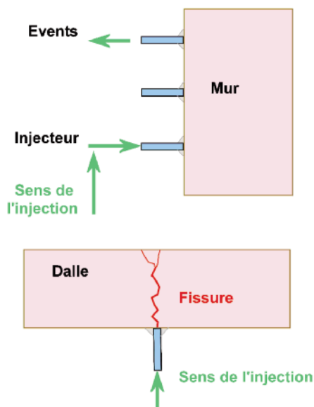
Figure n° 13 : exemples d'injection par l'évent le plus bas
